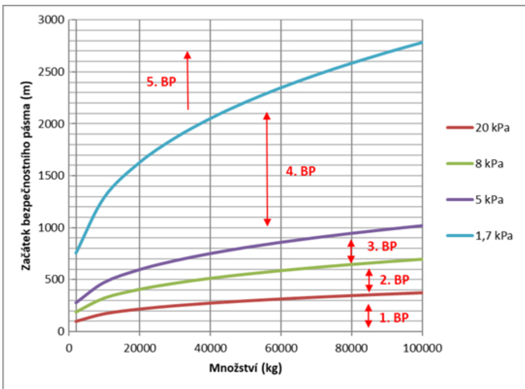
Obr. 1: Přetlak na počátečních hranicích jednotlivých bezpečnostních pásem v závislosti na množství výbuštiny třídy A
